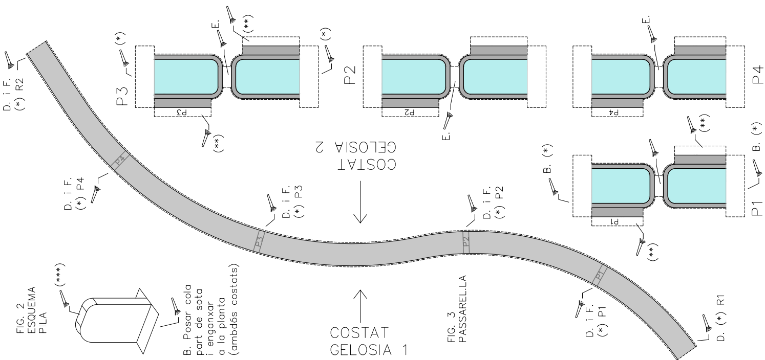
FIG. 1 ESQUEMA RAMPA
